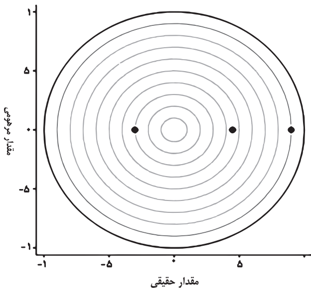
شکل ۳: آزمون ثبات (پایداری) مدل فقر، ارزش افزوده صنعت، و نابرابری
